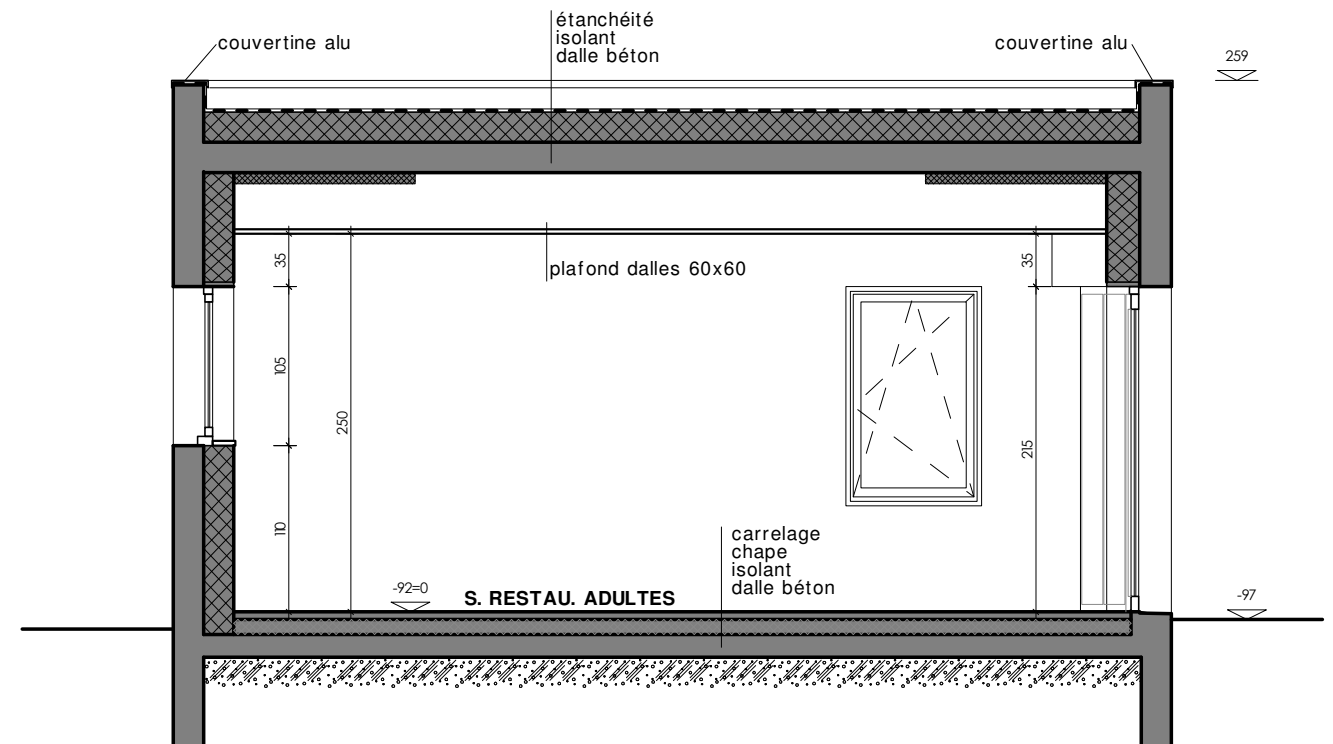
Coupe HH
