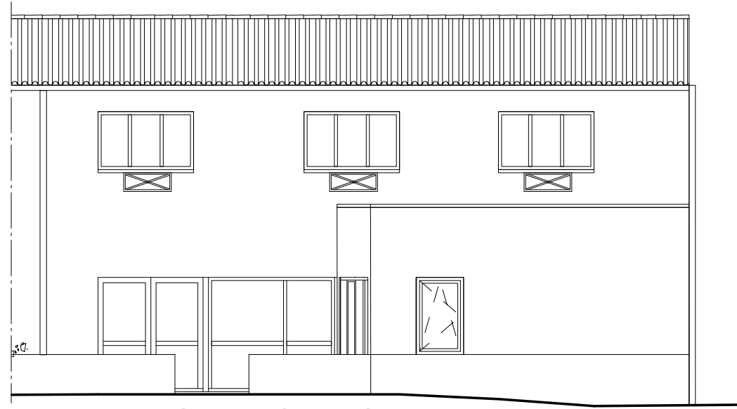
Façade SUD-OUEST
