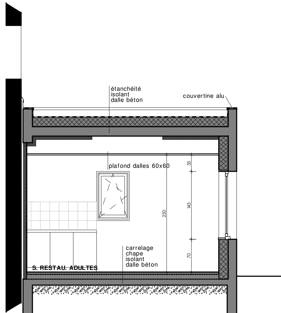
Coupe GG
